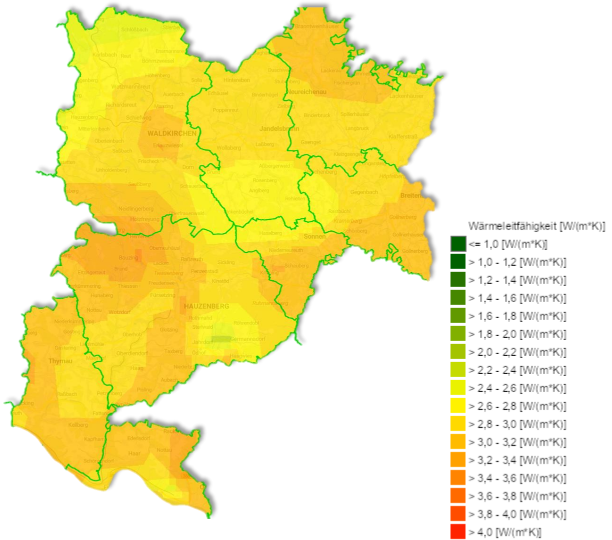
Abbildung 22: Mögliche Wärmeleitfähigkeit der ILE Abteiland; Quelle: Energieatlas Bayern
